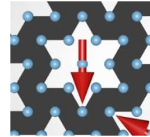
Magnet 1T\text{-TaS}_2
